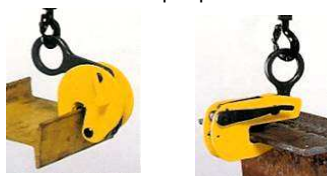
Pinze per profilati
